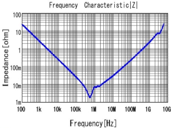
■ GRM32ER60J107ME20 |Z| DC0V, 25degC
