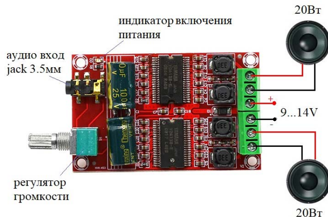
Эскиз подключения
