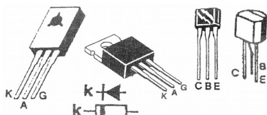
Рис.3 Цоколевка радиоэлементов
