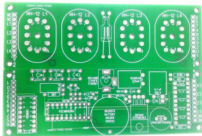
Монтажная схема
