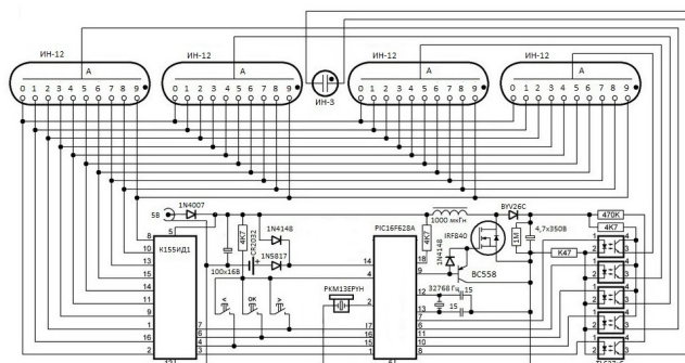
Электрическая схема
