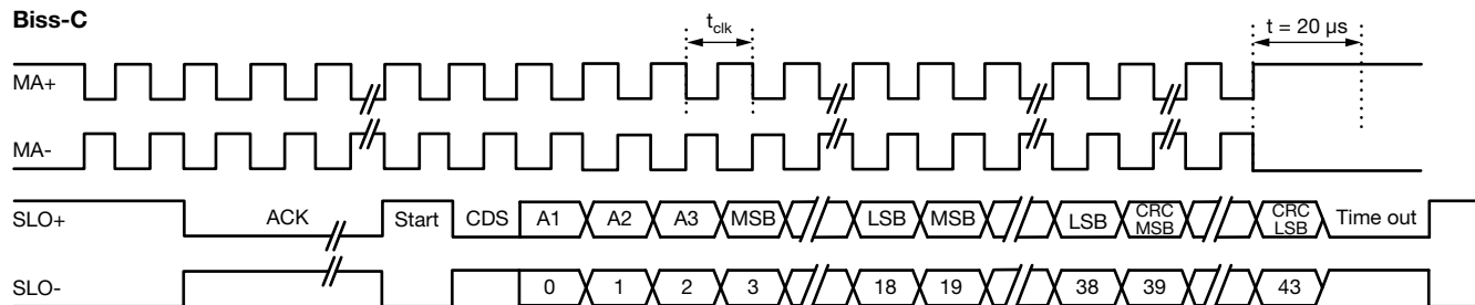
Fig. 4 - Biss-C Chronogram
