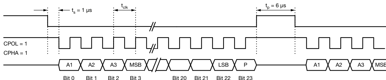
Fig. 5 - SPI Chronogram
