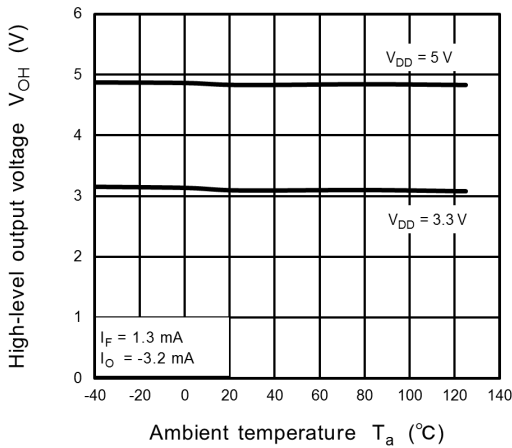
Fig. 12.2.6 V_{OH} - T_a
