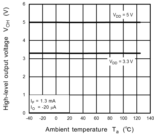
Fig. 12.2.5 V_{OH} - T_a
