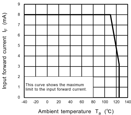
Fig. 12.2.2 I_F - T_a
