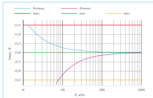
Рис. 6 (е). График зависимости для VDR160[...]15.
