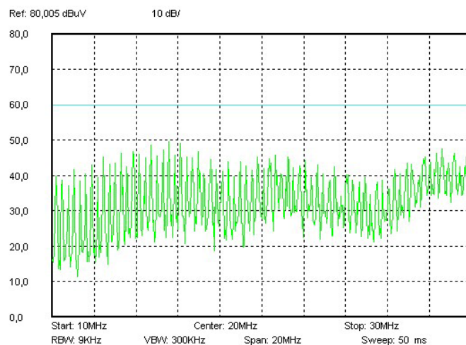
Рис. 12 (б). Спектрограмма 10–30 МГц.
