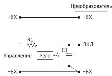
Рис. 4 (а). ВКЛ/ВЫКЛ с помощью реле.
