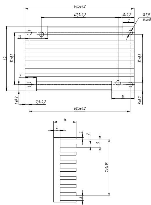
Рис. 15 (в).752695.263.
