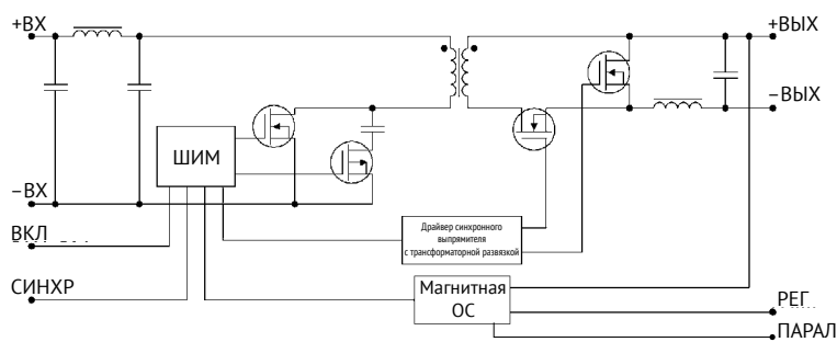
Рис. 1. Топология VDR160.
