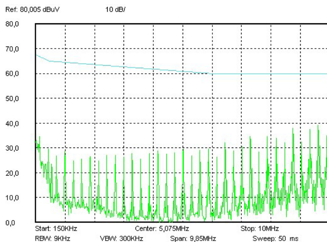
Рис. 12 (а). Спектрограмма 0,15–10 МГц.
