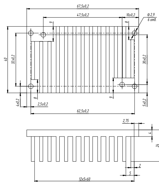
Рис. 15 (б).752695.055-01.
