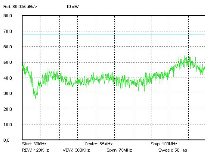
Рис. 12 (в). Спектрограмма 30–100 МГц.
