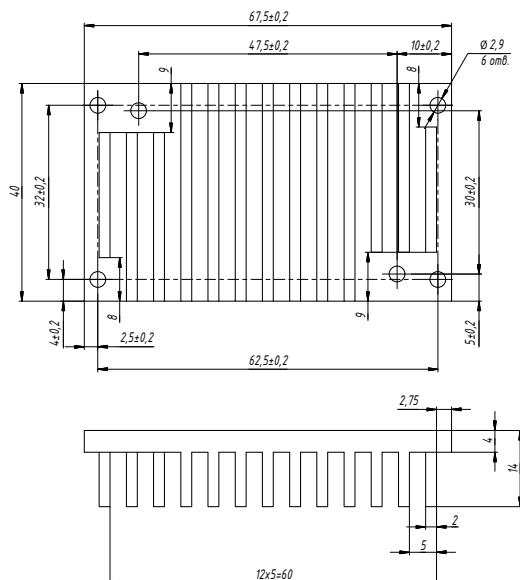
Рис. 15 (а).752695.055.
