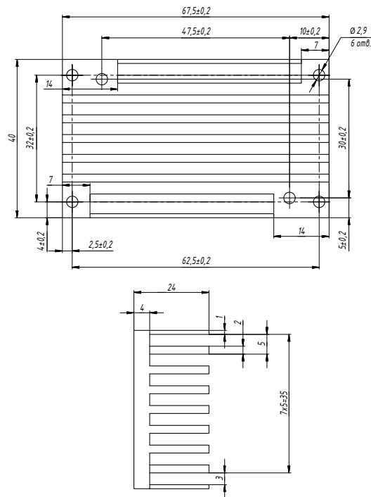
Рис. 15 (г).752695.263-01.
