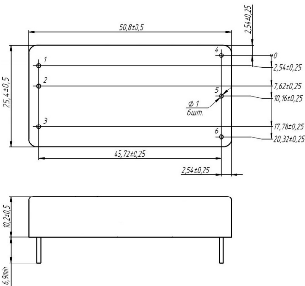
Рис. 5. Исполнение VDRI40, VDRI60.
