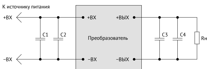
Рис. 2. Схема включения VDRI40, VDRI60.
