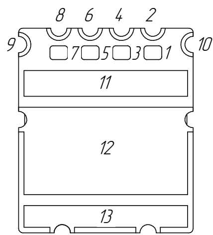
Рис. 2. Расположение выводов модуля EULER (вид снизу).
