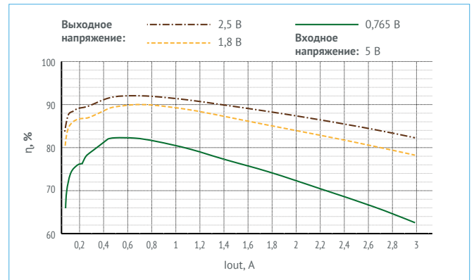
Рис. 13. V_{IN} = 5 \text{ В} ; V_{OUT} = 0,765 \text{ В} ; 1,8 \text{ В} ; 2,5 \text{ В} .
