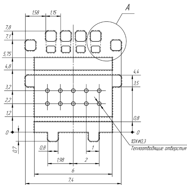
Рис. 24. Пример посадочного места на п/п (слой меди «пунтир. линия»/вскрытие маски «сплошная линия») / Land pattern example.
