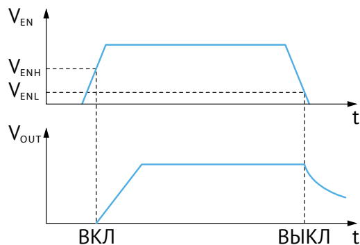
Рис. 14. ВКЛ/ВЫКЛ в зависимости от V_{EN}
