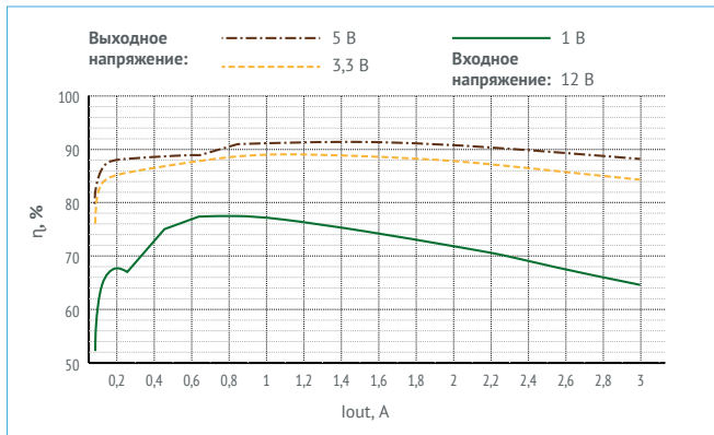
Рис. 12. V_{IN} = 12 \text{ В} ; V_{OUT} = 1 \text{ В} ; 3,3 \text{ В} ; 5 \text{ В} .
