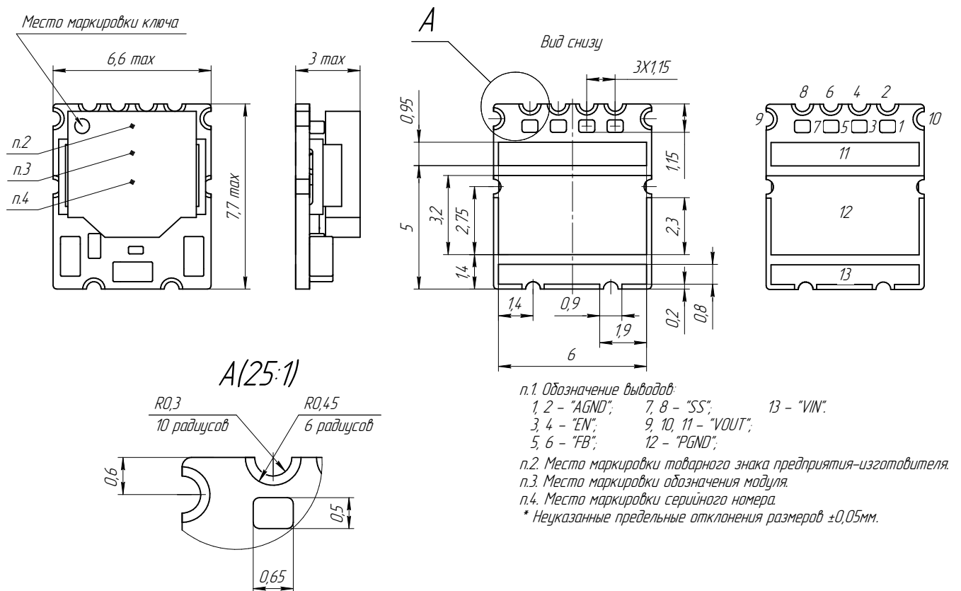
Рис. 21. Габаритный чертёж
