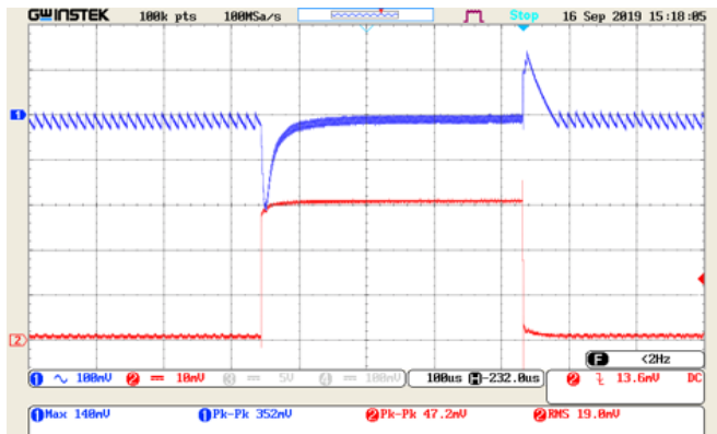
Рис. 7. I_{OUT} = 0,1-3 \text{ A} ; 6,5 \text{ A/мкс.}
