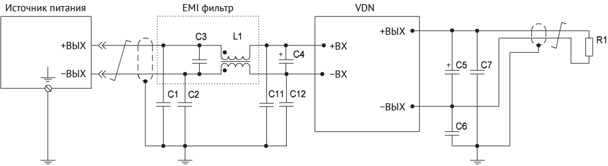
Рис. 2. Типовая схема подключения.
