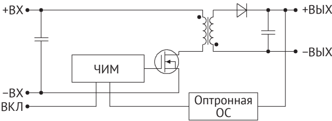
Рис. 1. Топология VDN5.
